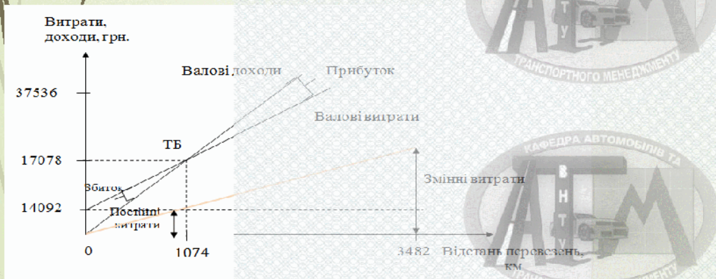
Графік беззбитковості для маршруту запропонованим рухомим складом
