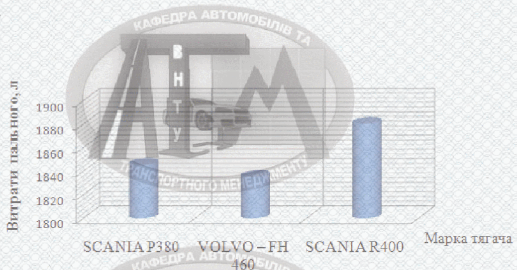
Рисунок 3.2 – Витрати пального на оборотний рейс за марками сідельних тягачів
