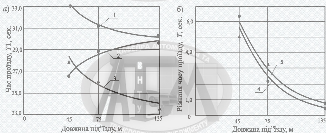
а) час проїзду автомобіля зони впливу; б) різниця часу проїзду зони впливу “пов'язаними” і “вільними” автомобілями
