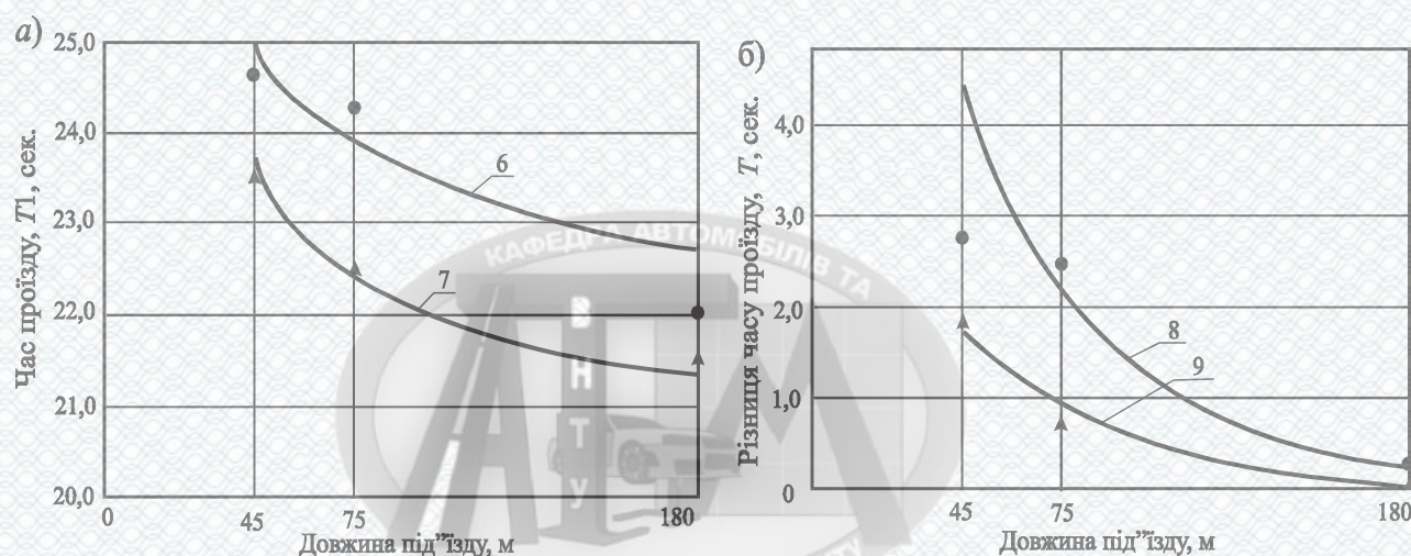
а) час проїзду зони впливу “пов’язаними” автомобілями; б) різниця часу проїзду зони впливу “пов’язаними” і “вільними” автомобілями
