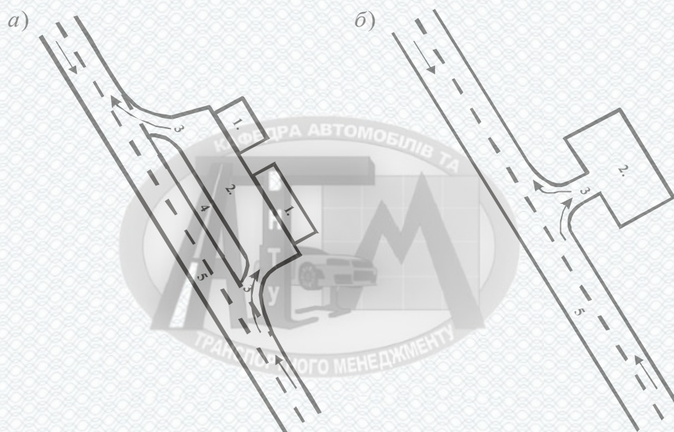
а) фронтальна; б) тупикова. 1 – споруда; 2 – стоянка; 3 – під'їзди; 4 – газон; 5 – основна дорога.
