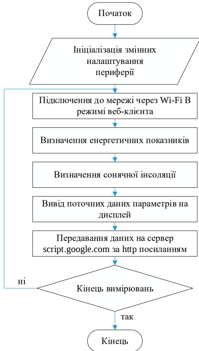
Рисунок Г.4 – Алгоритм мікроконтролера
