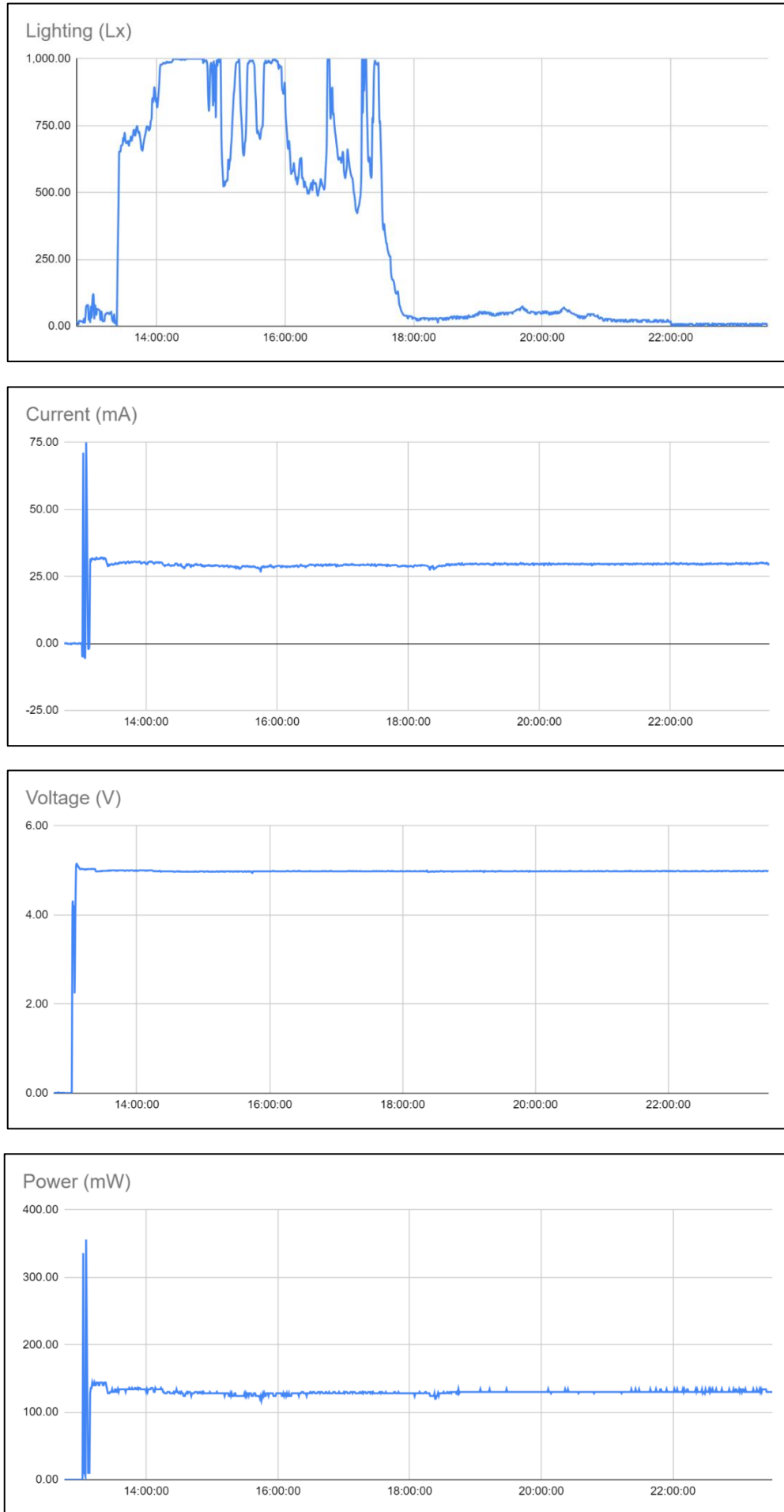
Рисунок Г.6 – Графіки тестування IoT-системи
