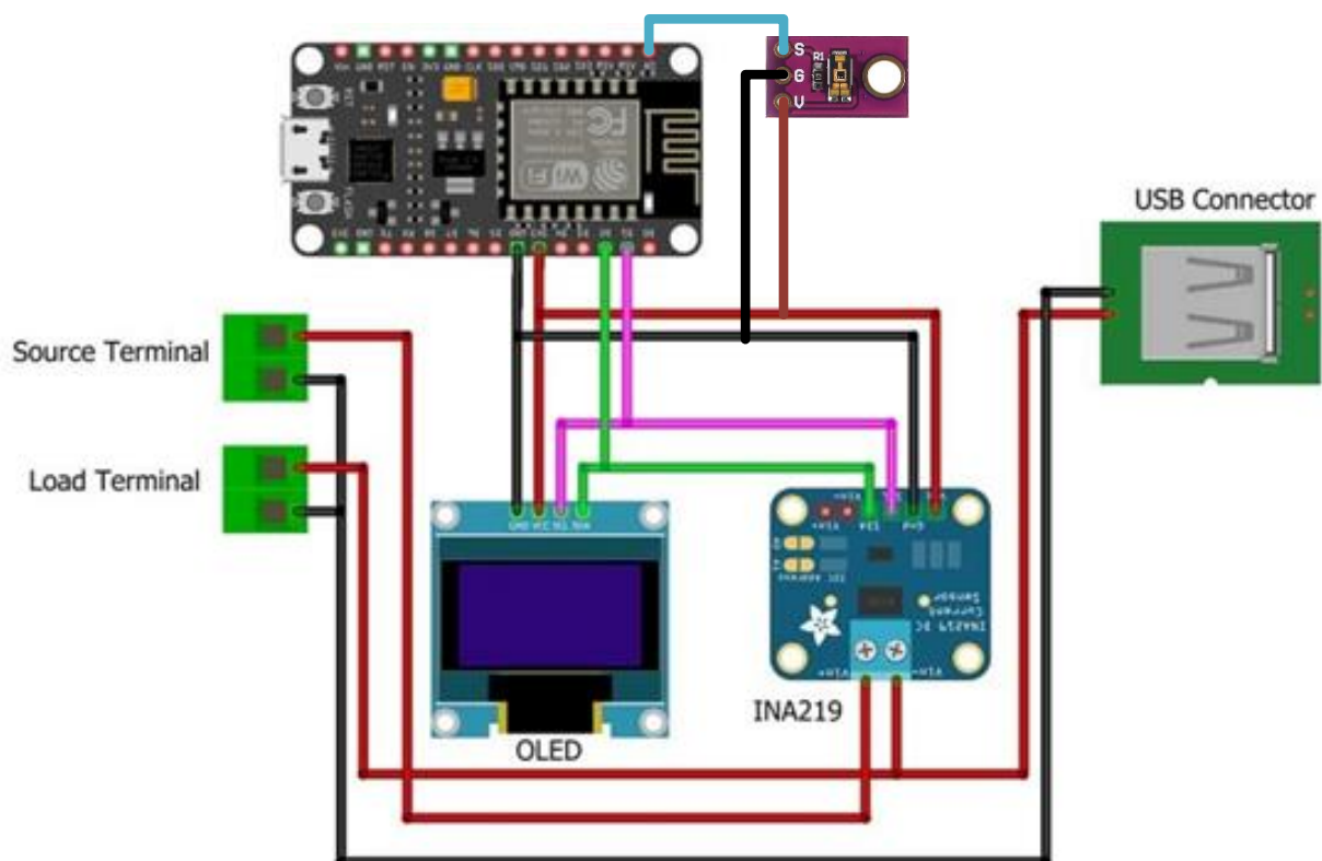
Рисунок 4.1 – Схема IoT пристрою для аналізу генерації електроенергії фотоелектричними модулями
