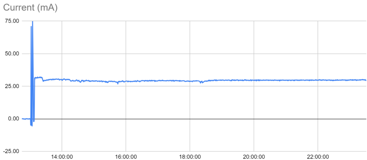
Рисунок 4.5 – Графік струму одержаний в тестовому режимі
