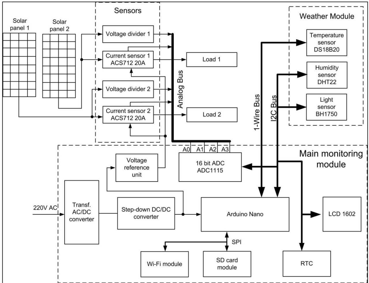
Рисунок Г.2 - Структурна схема пристрою моніторингу генерації сонячної панелі
