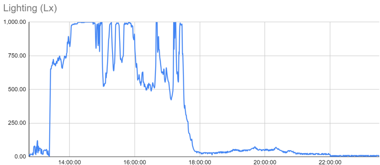
Рисунок 4.4 – Графік освітленості одержаний в тестовому режимі
