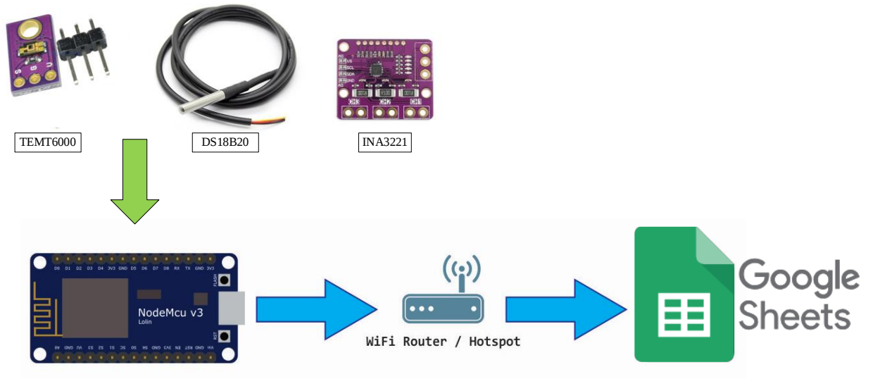
Рисунок Г.3 - Структурна схема IoT-системи оцінювання ефективності функціонування фотоелектричних модулів
