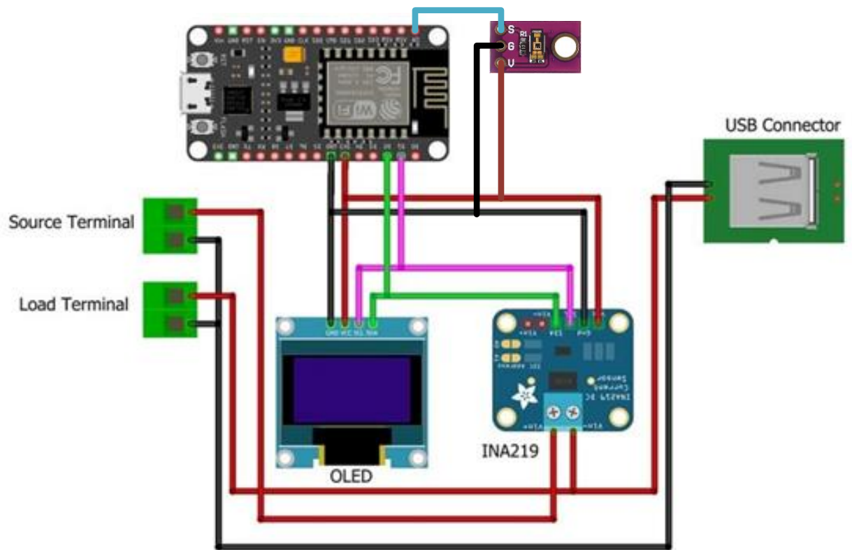
Рисунок Г.5 - Схема IoT пристрою для аналізу генерації електроенергії фотоелектричними модулями
