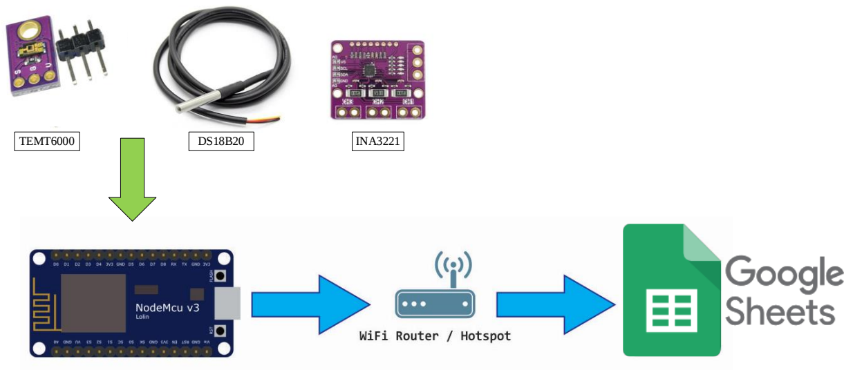
Рисунок 3.2 - Структурна схема IoT-системи оцінювання ефективності функціонування фотоелектричних модулів
