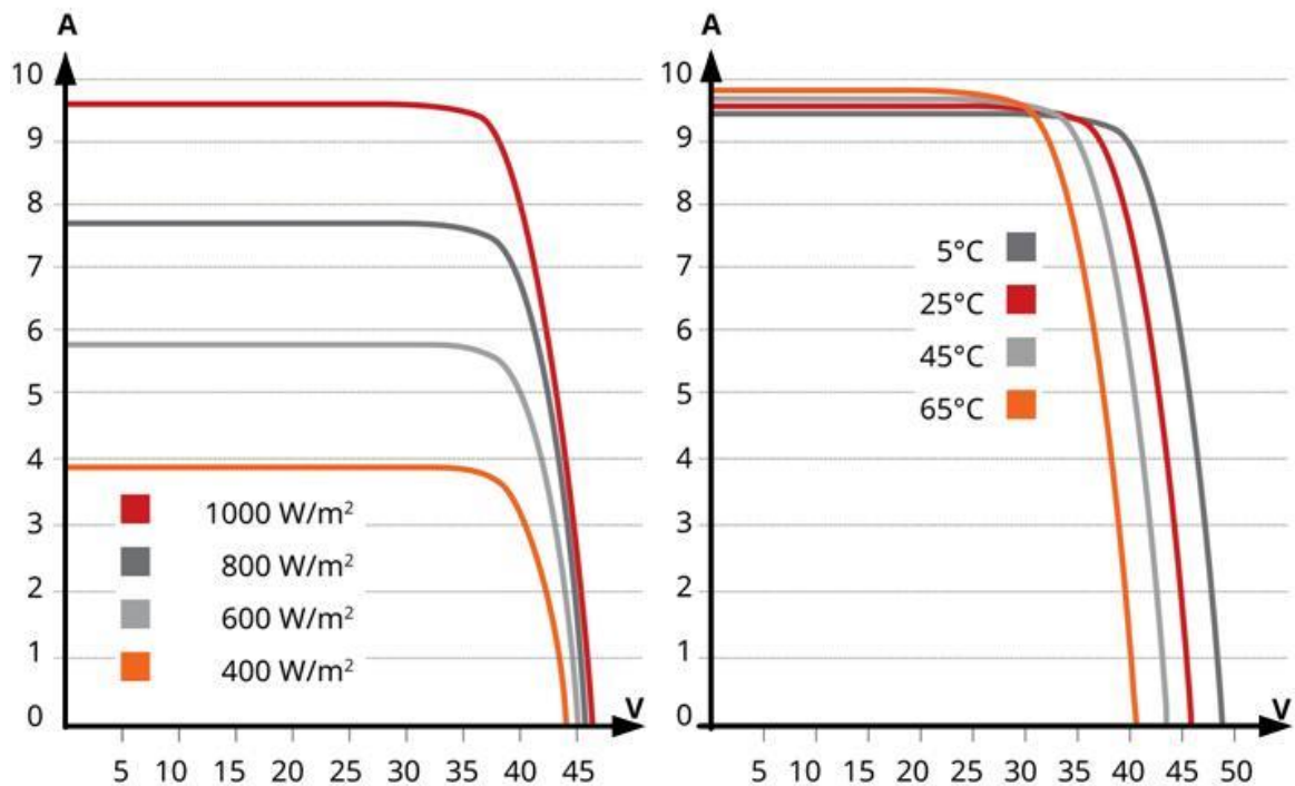
Рисунок 2.3. Вольт-амперні характеристики сонячної панелі MAXPOWER CS6U-345P
