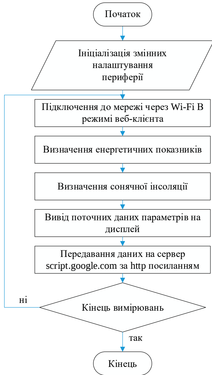
Рисунок 3.7 – Алгоритм мікроконтролера
