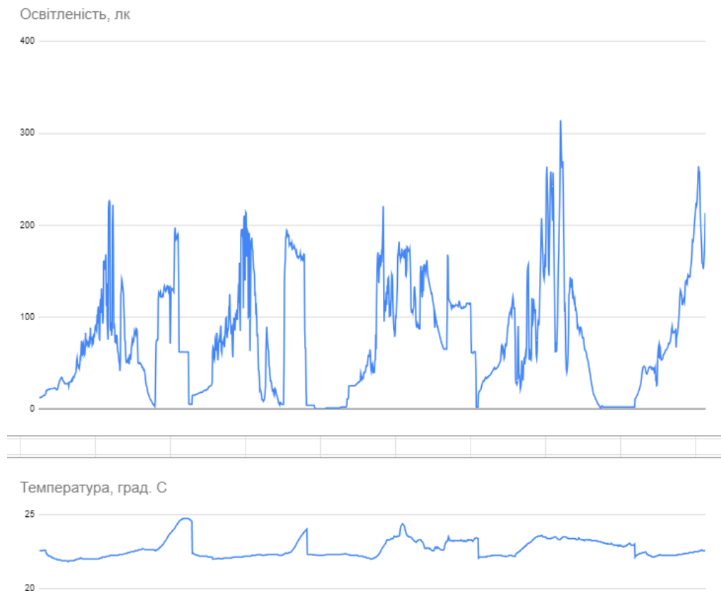
Рисунок 3.18 – Графіки зміни освітленості та температури на протязі 5-денного періоду спостережень
