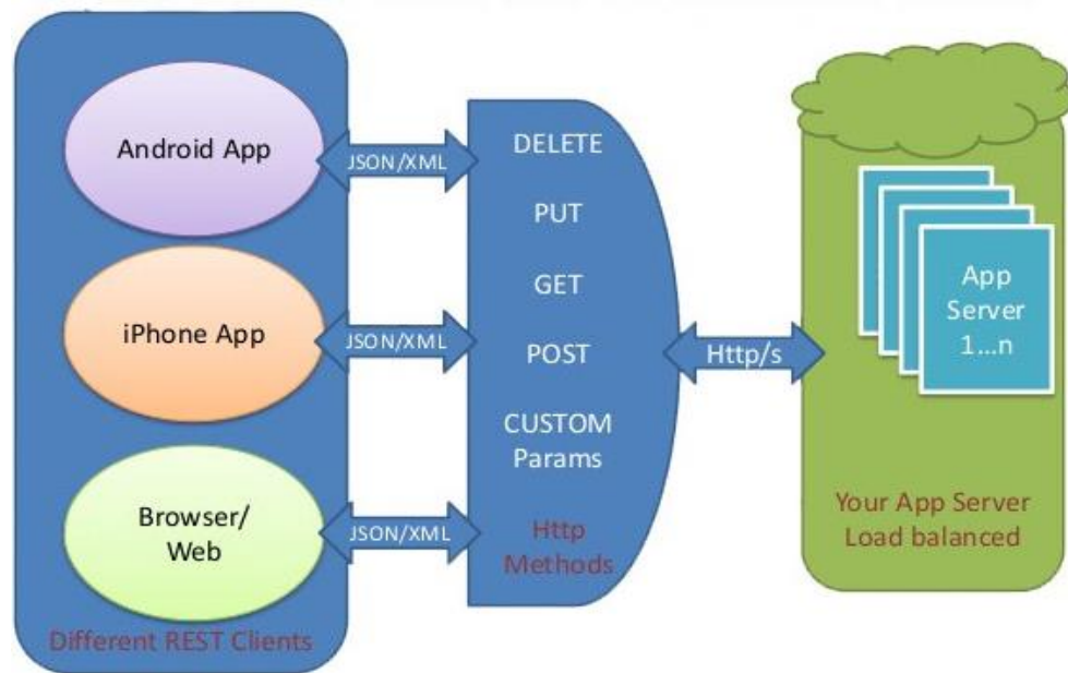
Рисунок 3.3 – Алгоритм роботи REST API
