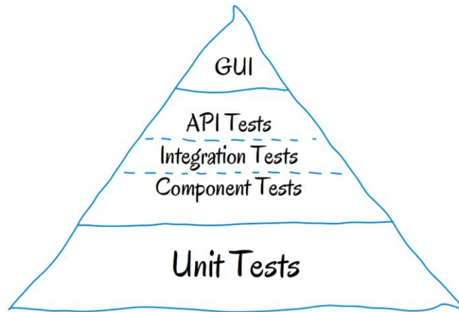
Рисунок 2.1 - Піраміда тестів
