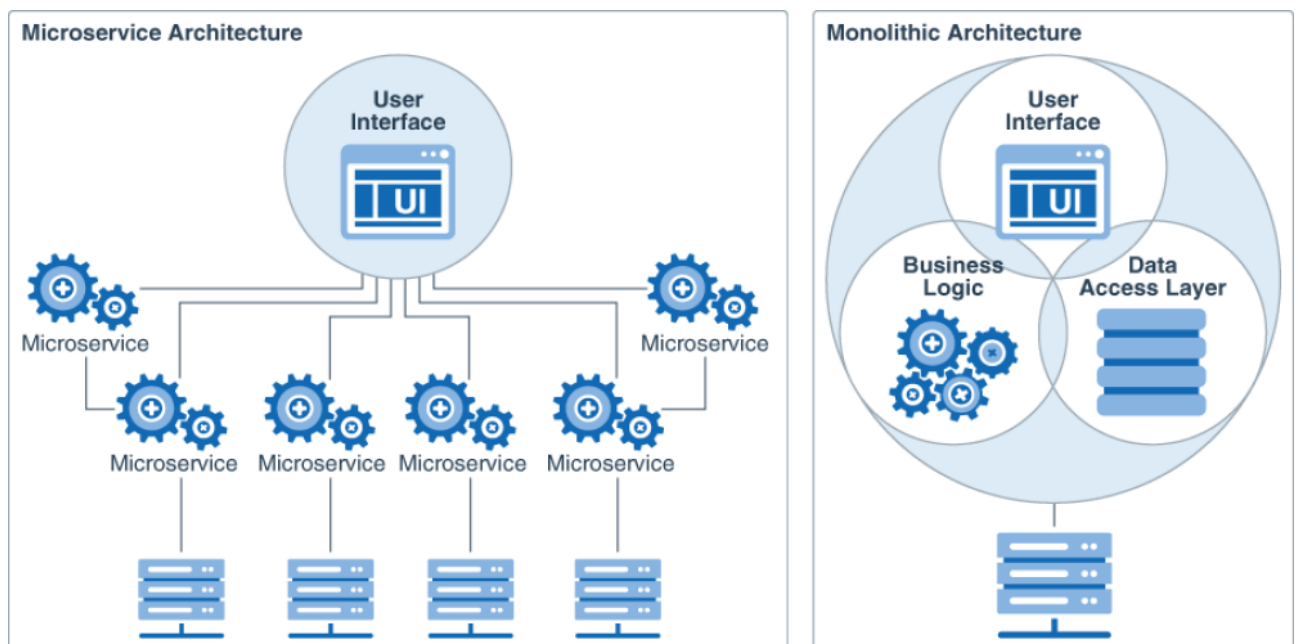
Рисунок 3.1 - Схема різних архітектурних типів
