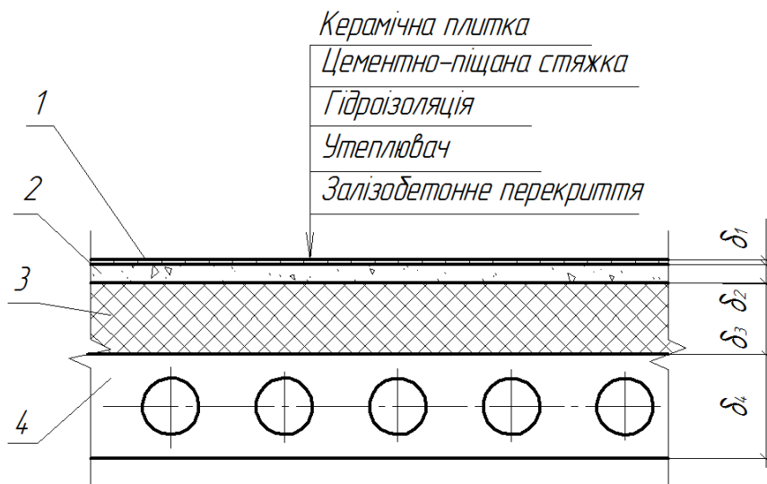
Рис. 2.3 – Конструктивна схема підлоги до теплотехнічного розрахунку
