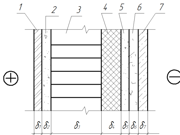
Рис. 2.2 – Конструктивна схема стіни до теплотехнічного розрахунку.
