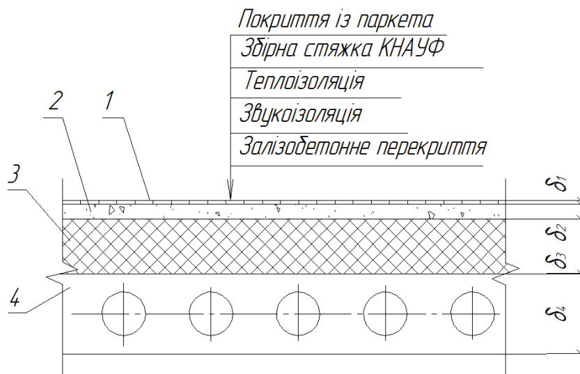
Рис. 2.4 – Конструктивна схема підлоги до теплотехнічного розрахунку
