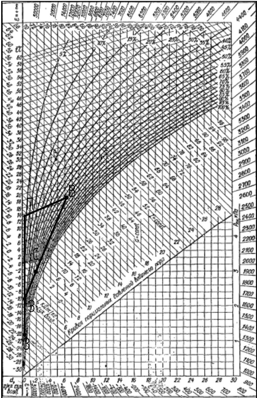
Рис. Е.2 - Схема обработки воздуха в холодный период року для приміщення спортзалу
