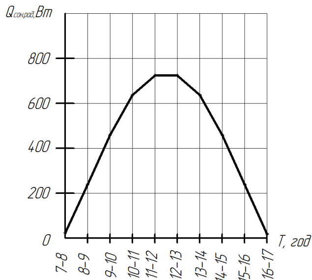
Рис. 2.6 - Графічна залежність енергетичної освітленості площин для півдня сонячною радіацією у січні за умов ясного неба.
