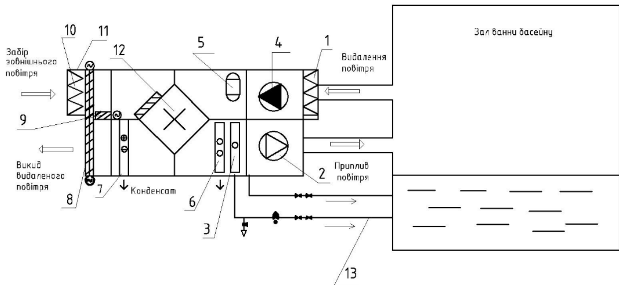
Рис. 2.7 - Схема роботи вентиляційної установки з рекуператором з утилізацією вологи:
