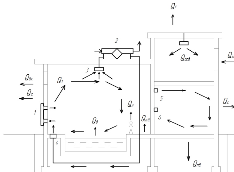
Рис. 2.1 - Розрахункова схема до моделювання теплового розрахунку будівлі:
