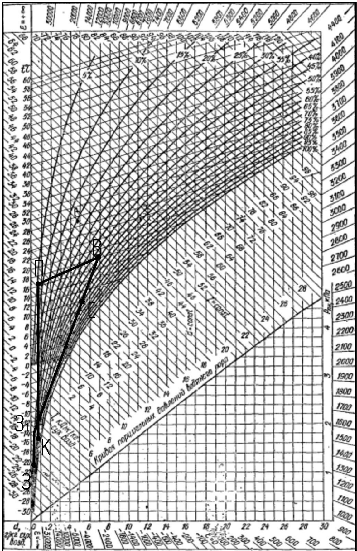
Рис. Е.4 - Схема обработки воздуха в холодный период року для помещения музыкального зала та групповой комнаты №19
