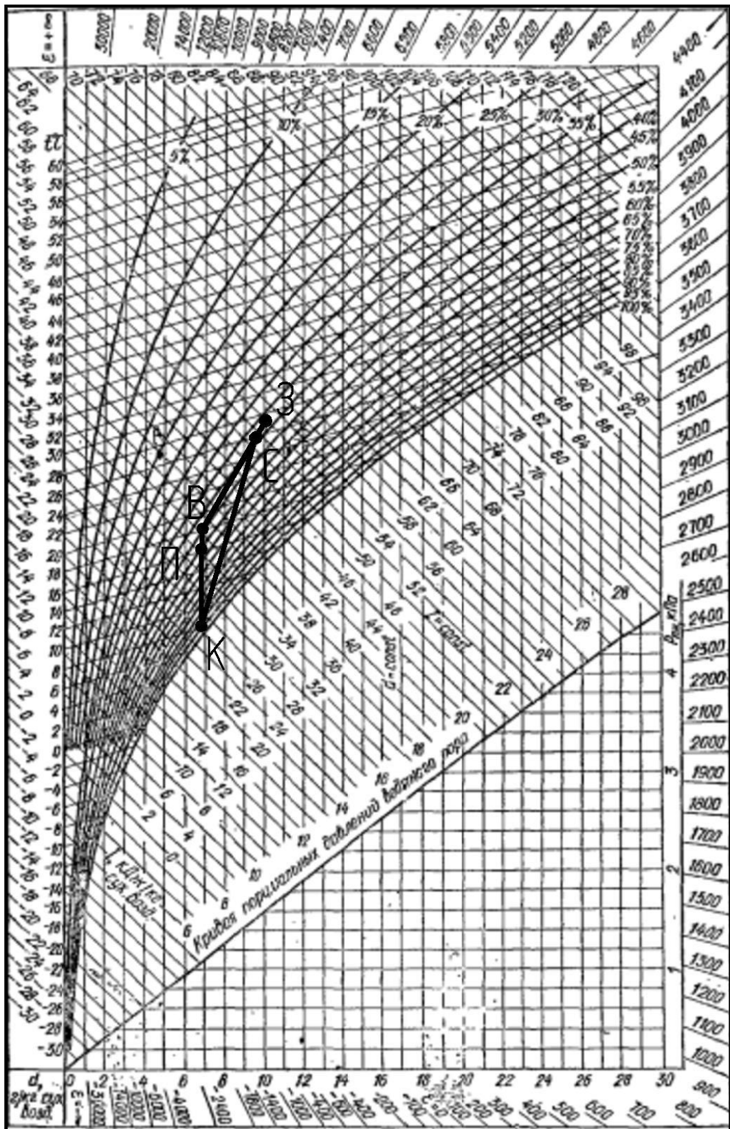
Рис. Е.5 - Схема обработки воздуха в теплый период року для помещений кабинетів
