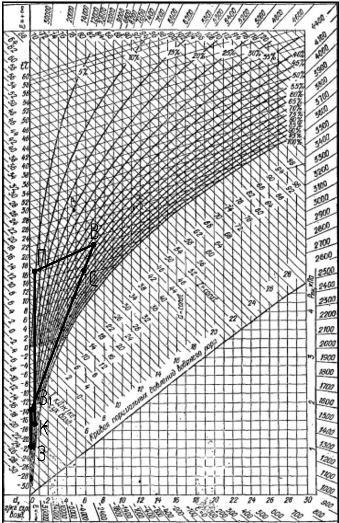
Рис. Е.6 - Схема обработки воздуха в холодный период года для помещений кабинетів
