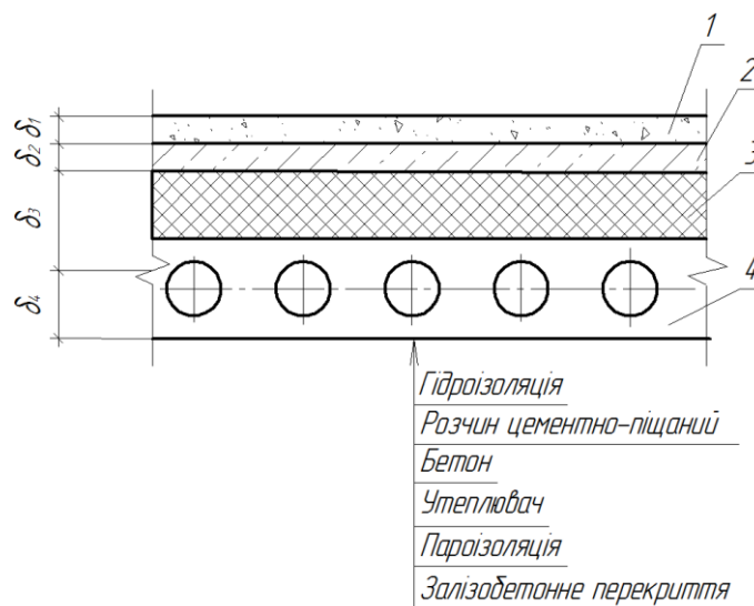
Рис. 2.5 – Конструктивна схема горища до теплотехнічного розрахунку.
