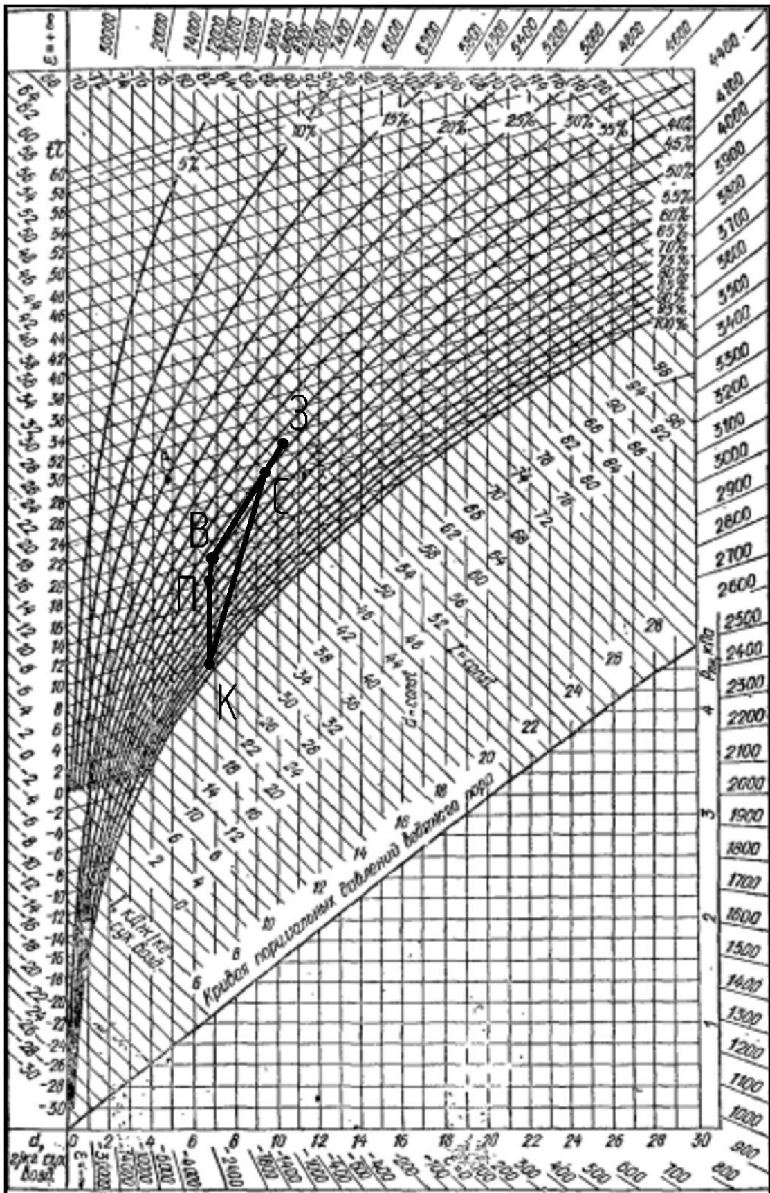
Рис. Е.3 - Схема обработки повітря в теплий період року для приміщення музичного залу та групової кімнати №19
