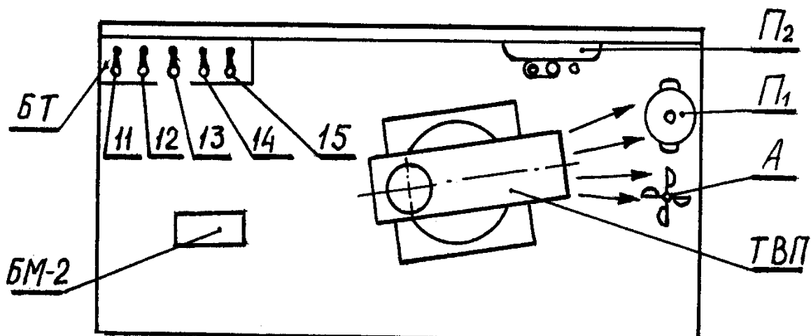
Рисунок 9.3 – План розміщення приладів та ТВП на лабораторному столі
