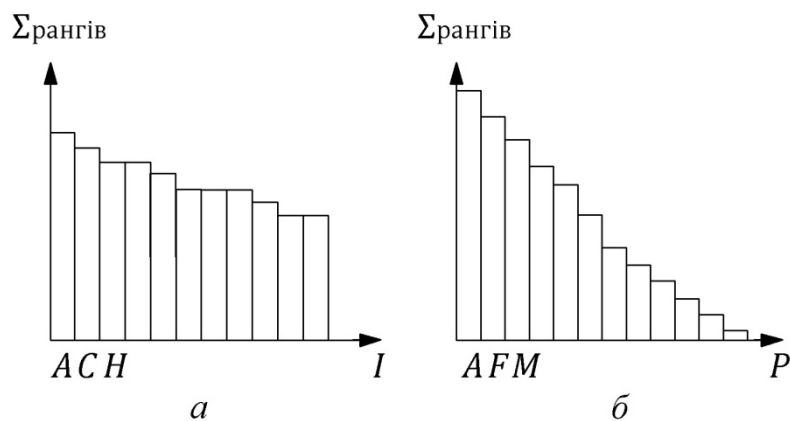
Рисунок 3.7 – Діаграма рангів: а – за рівномірного розподілу рангів; б – за нерівномірного розподілу рангів
