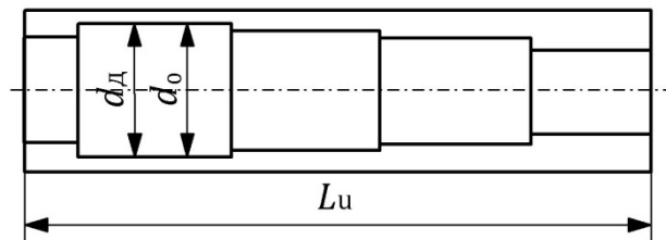
Рисунок 4.19 – Ескіз деталі
