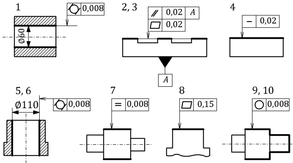
Рисунок 4.16 – Варіанти форми поверхонь деталей
