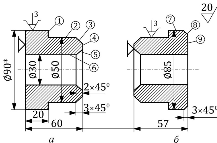
Рисунок 4.9 – Схема токарного оброблення деталі: a – установлення А; б – установлення Б
