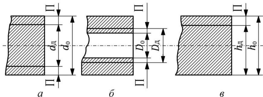
Рисунок 4.6 – Загальне припускання на механічне оброблення: a – зовнішня поверхня обертання; б – внутрішня поверхня обертання; в – плоска поверхня
