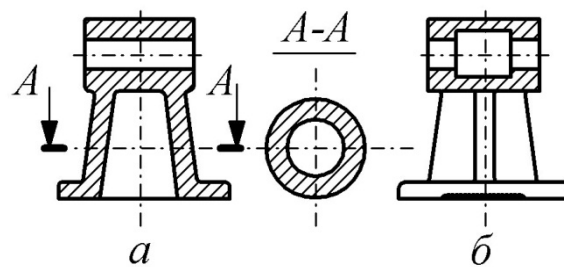
Рисунок 4.13 – Ескіз деталі: a – перший варіант конструкції; б – другий варіант конструкції
