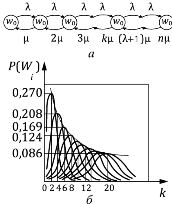
Рисунок 6.1 – Стан складської системи за ступенем завантаженості зони зберігання транспортними партіями вантажів: а – розмічений граф станів; б – графіки розподілу кількостей транспортних партій, що фактично зберігаються
