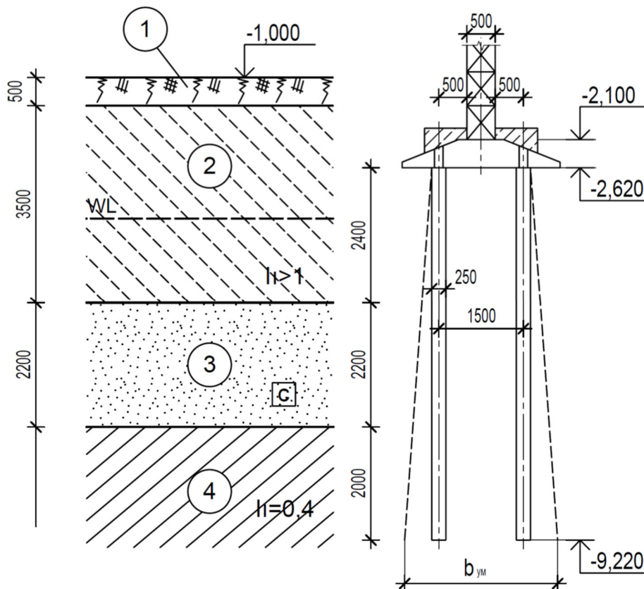
Рисунок 27 – Положення буроін'єкційних паль підсилення у ґрунті
