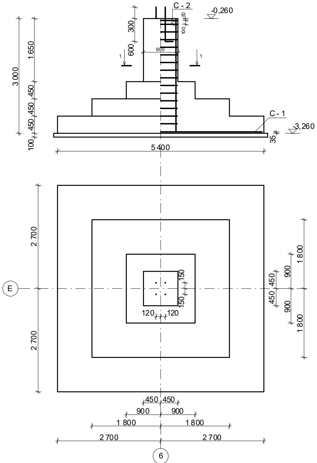
Рисунок 8 – Конструктивне рішення фундаменту мілкого закладання
