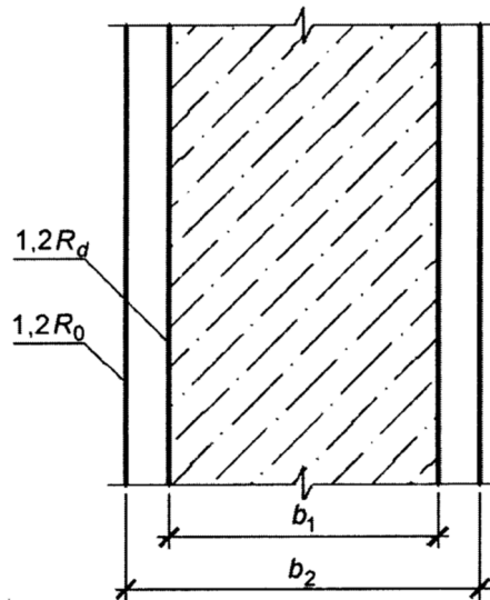
Рисунок 24 – Обмеження тисків під подошвою стрічкових фундаментів
