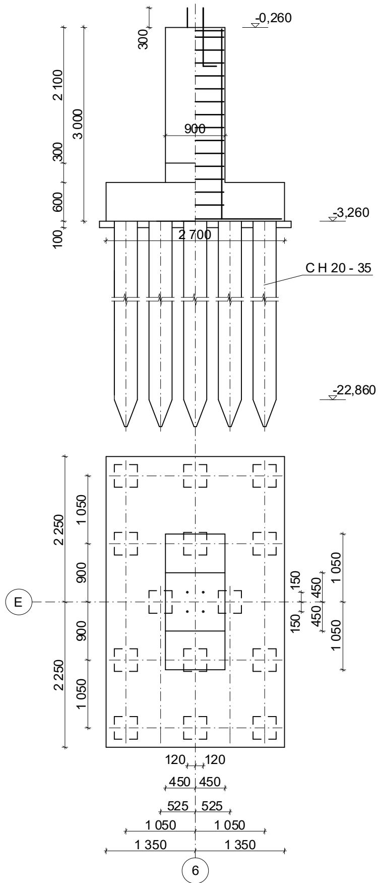
Рисунок 9 – Конструкція фундаменту у варіанті із забивних паль
