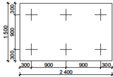
Рисунок 15 – Розмір підосви ростверку в плані
