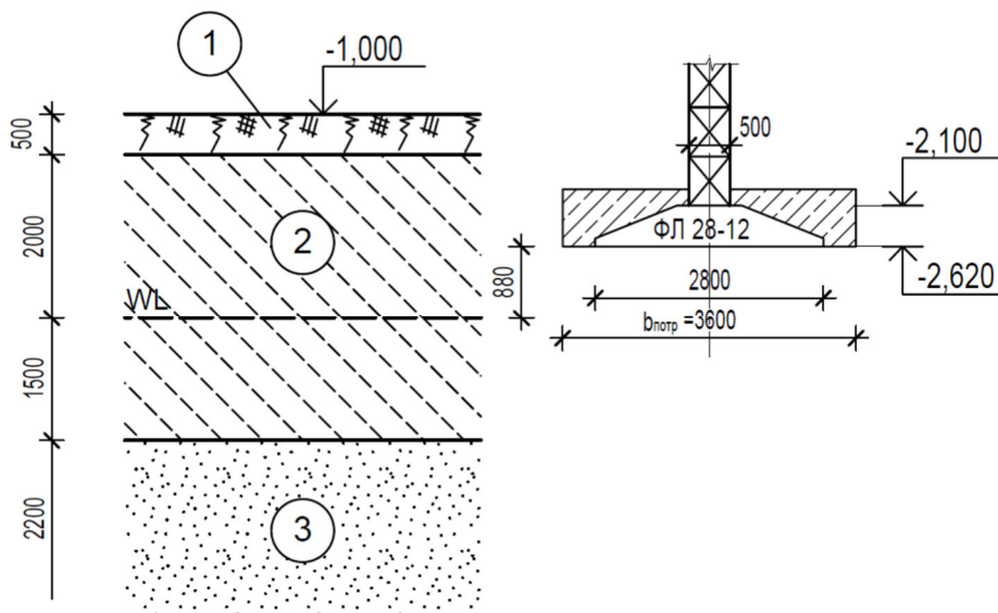
Рисунок 26 – Положення фундаментів мілко закладання, підсилених банкетами, у ґрунті
