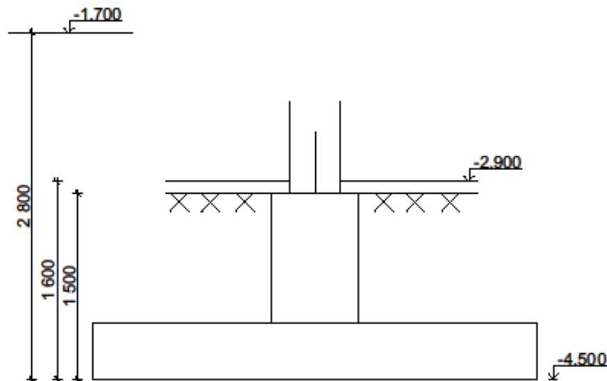
Рисунок 14 – Положення фундаменту мілкового закладання і ростверку пального фундаменту у ґрунті
