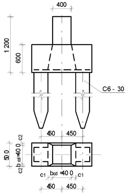
Рисунок 22 – Конструктивне рішення і розрахункова схема ростверку для забивних паль
