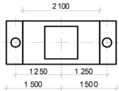
Рисунок 31 - Розміщення палей підсилення в плані
