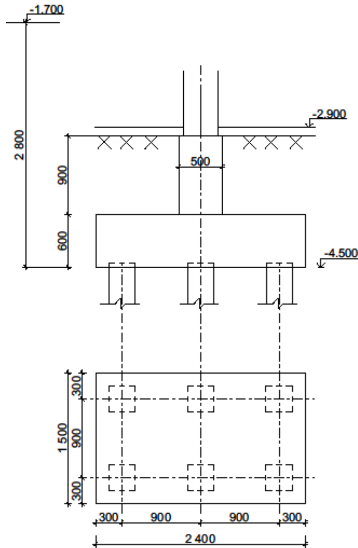
Рисунок 17 – Конструктивне рішення ростверку пальового фундаменту під монолітну залізобетонну колону
