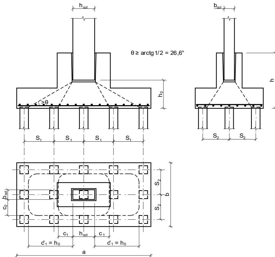
Рисунок 18 – Схема утворення пірамід продавлювання від дна стакану під збірною залізобетонною колоною при багаторядному розміщенні паль
