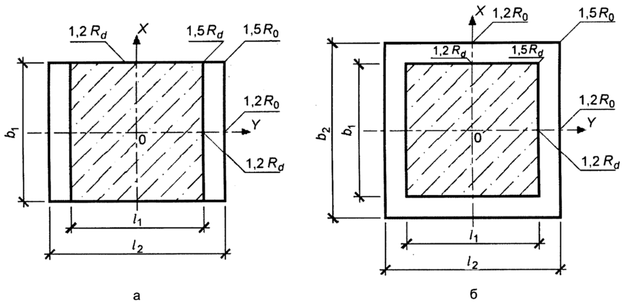
Рисунок 23 – Обмеження контактних тисків для стовпчастих фундаментів
