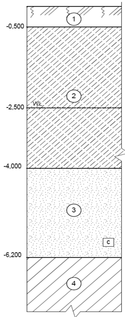
Рисунок 25 – Інженерно-геологічний розріз будівельного майданчика
