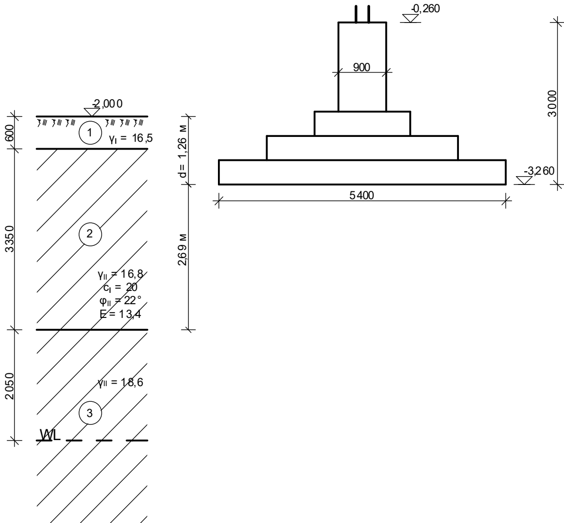
Рисунок 6 – Положення фундаменту мілкого закладання у ґрунті
