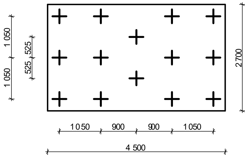
Рисунок 7 – Розміщення палів в плані у ростверку
