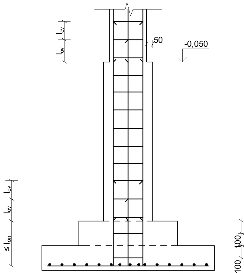
Рисунок 1 – Конструкція фундаменту під монолітну колону
