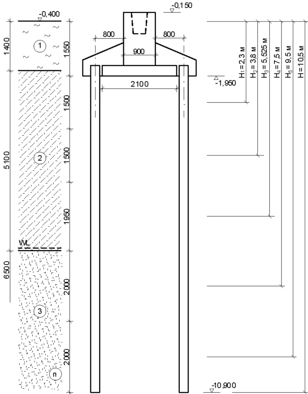
Рисунок 30 – Положення буроін'єкційних паль у ґрунті
