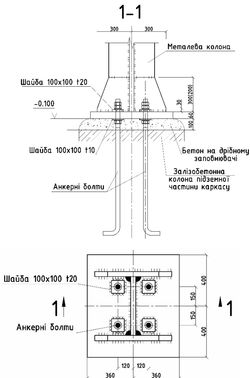
Рисунок 4 – Вузол обпирання металевої колони на підколоник
