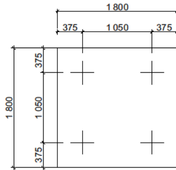
Рис. 11 - Розміри підшови ростверку в плані
