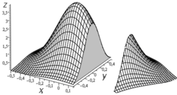
Рисунок 4 – Відсікання частини піксела, що має об'єм V(d) \Delta l(d)
