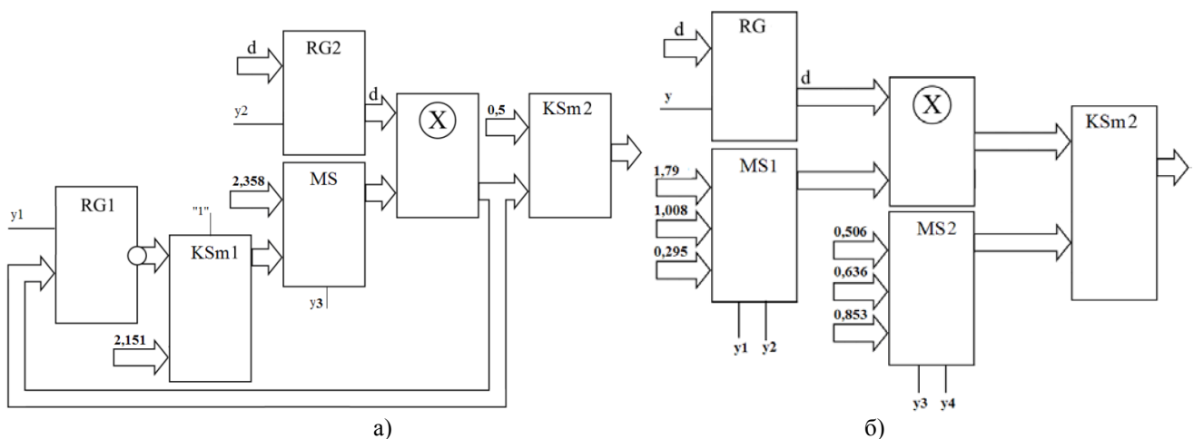
Рисунок 6 – Структурна схема обчислювального блоку розрахунку V(d) поліномами P_2(d) (а) і P_1(d) (б)
