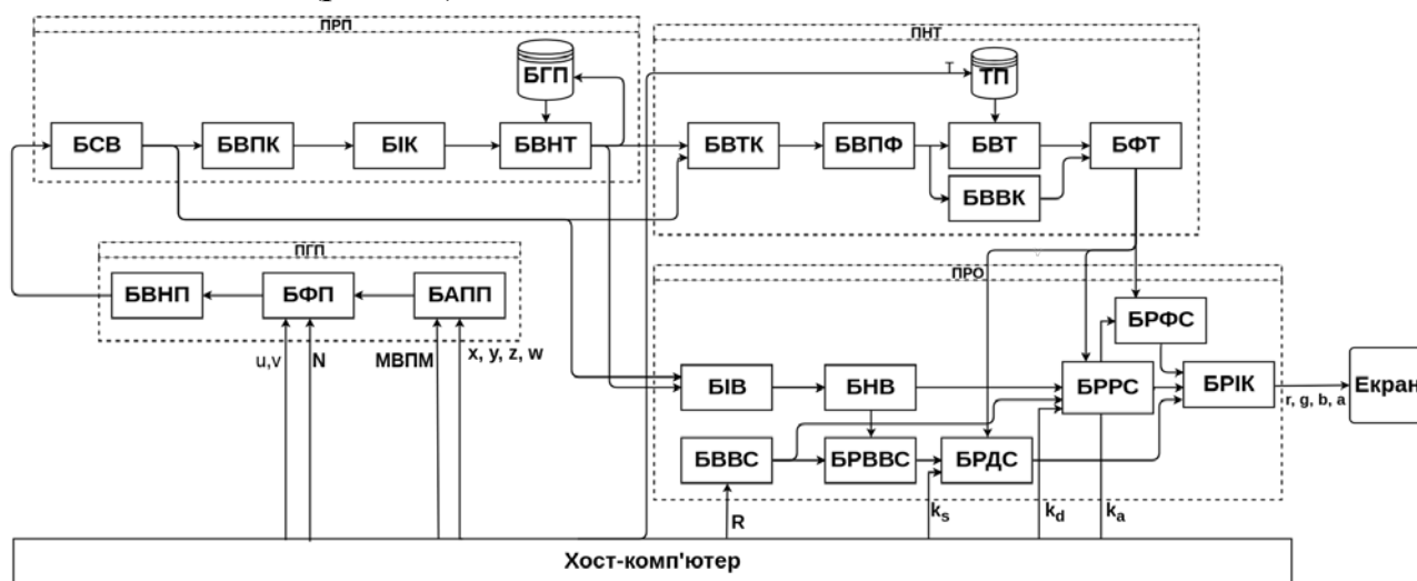
Рисунок 27 – Структурна схема системи кінцевої візуалізації
